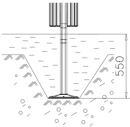
DET 4
