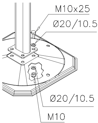
DET 5
