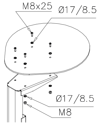
DET 6
